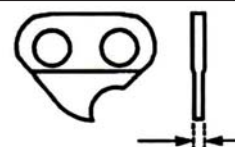
Eslabones de 56 ACC a 78 ACC
